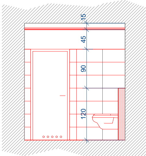
KŁAD 3-3
