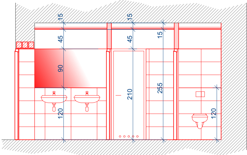
KŁAD 4-4
