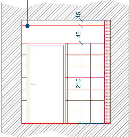
KŁAD 4-4
