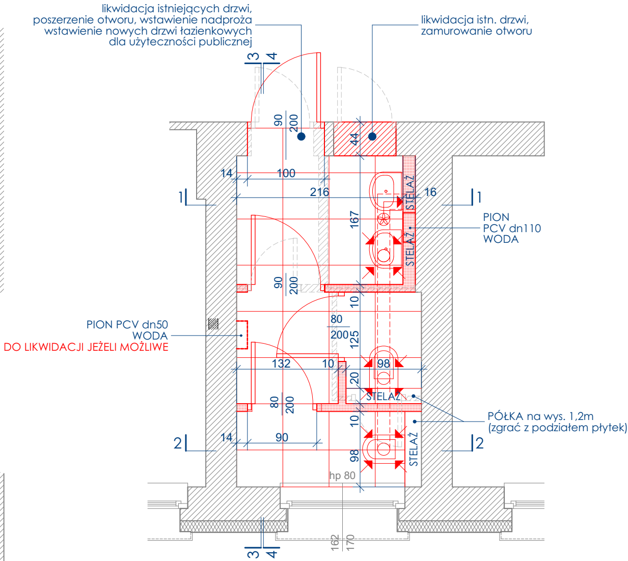
RZUT
