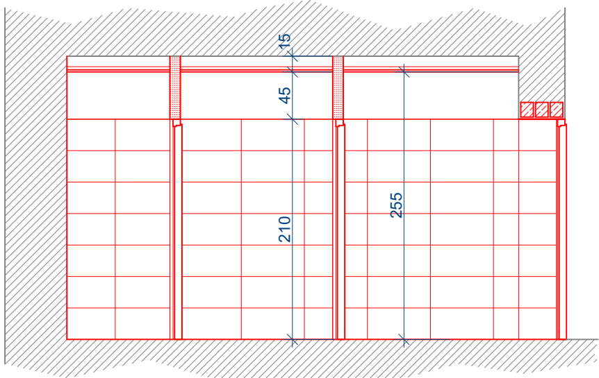
KŁAD 3-3
